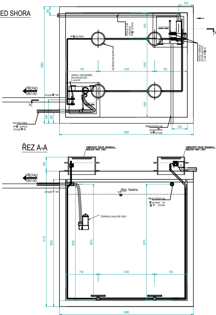
POHLED SHORA
